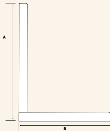
Poleia Soldada PCL 305
